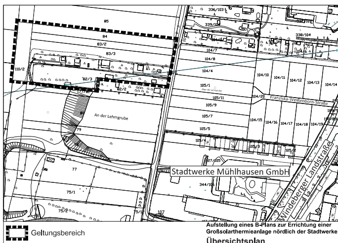
Übersichtsplan Geltungsbereich des vorhabenbezogenen Bebauungsplans Nr. VEP-36 "Solarpark Schröterode"
